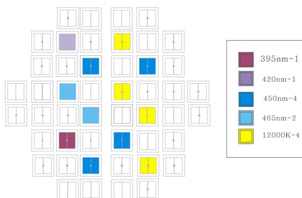
Fig. 1: Qube 30
