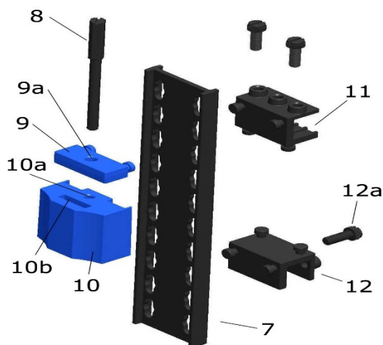
Rys. 3: Uchwyt EVO 501
